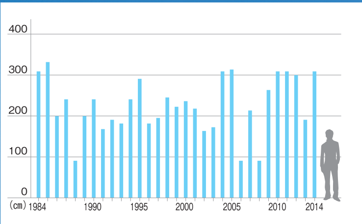
全年最大积雪深度图表(1984~2014)
